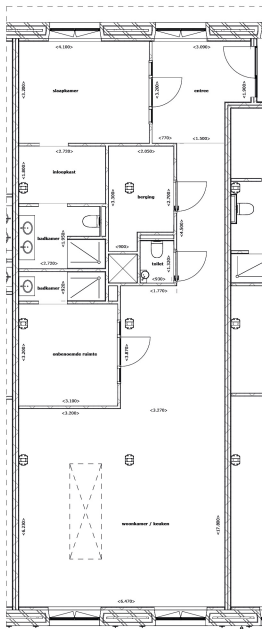
Plattegrond verdieping 02 1:50
